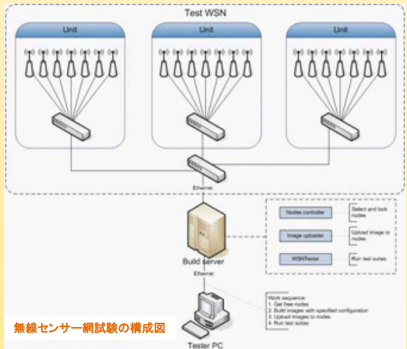
無線センサー網試験設備の一部
